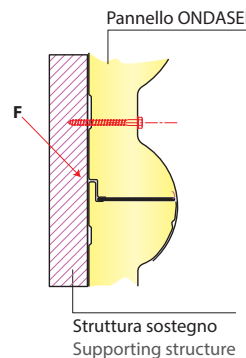
Montaggio orizzontale Horizontal mounting
